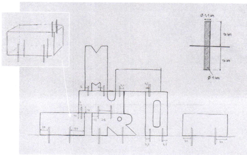
imatge 6. Sistema de ancoratge mitjançant barres i cotes proposades.
